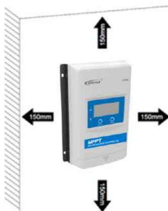
Рисунок 2-1 Монтаж
